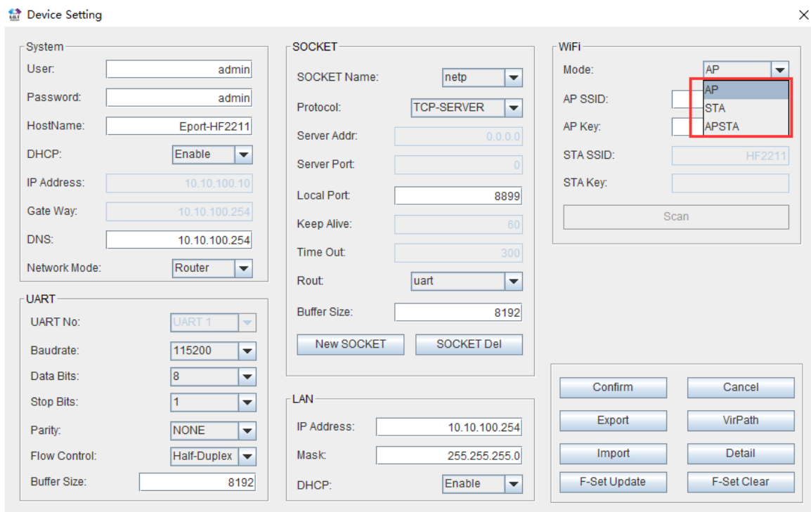
Figure 25. Configure Wi-Fi Parameter
